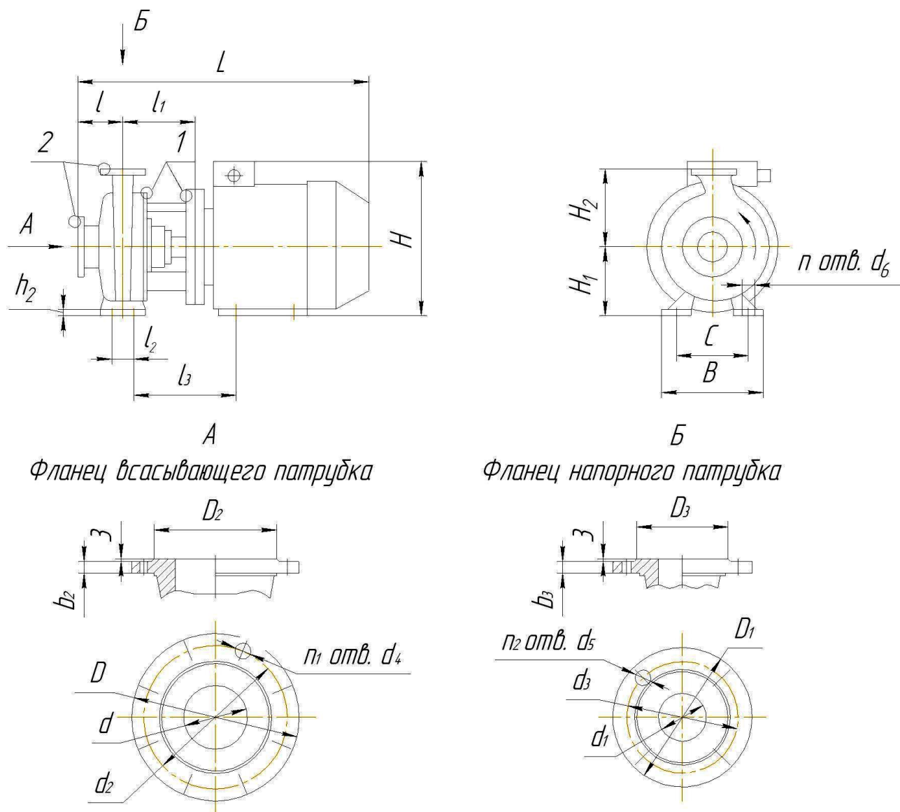
Рисунок 6 Габаритные и присоединительные размеры насосов типа «ХМ»
